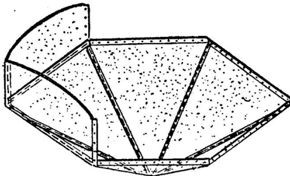
Fig. 6— COMPLETANDO LA PANTALLA
