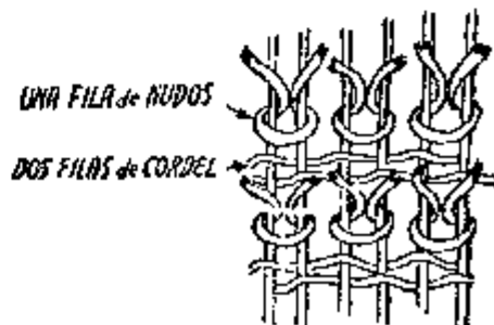
13 DIAGRAMA DEL TEJIDO
